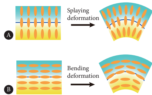
图 10 取向场失稳模式
