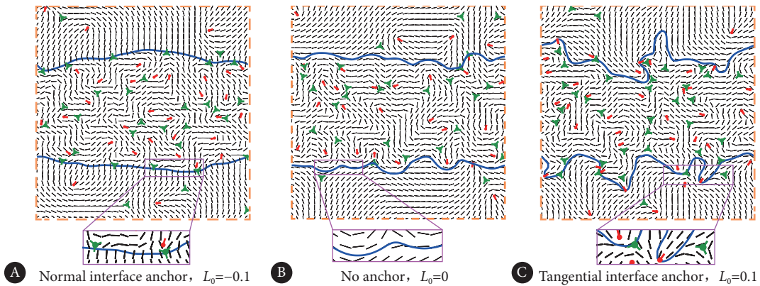
图 7 三种界面处的取向场及缺陷分布
