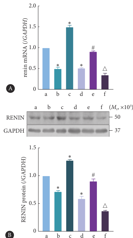
图5 1,25(OH) _2 D _3 通过与PKA 通路竞争来抑制肾素在蜕膜腺上皮细胞中的表达
