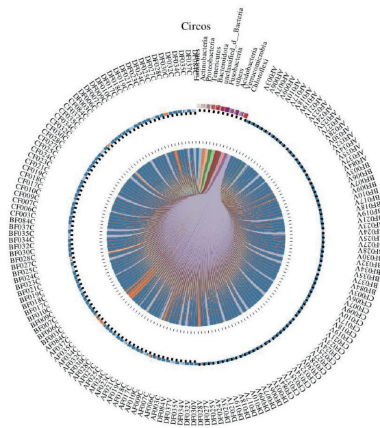
图 2 门水平基因组circos图 Fig 2 Genome circos map at the phylum level
